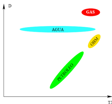
Figura 8: Grafico de interpretación de mapas de difusión mostrando zonas que permiten discriminar fluidos de igual T2 pero diferente difusión
