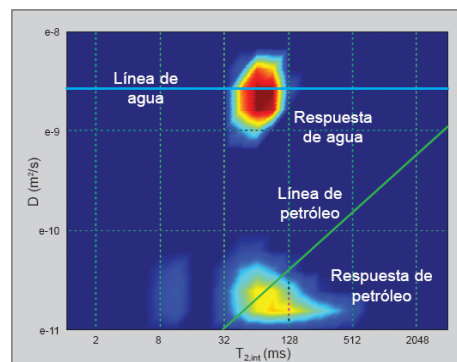
Figura 8: Grafico de interpretación de mapas de difusión mostrando zonas que permiten discriminar fluidos de igual T2 pero diferente difusión
