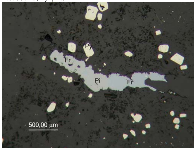
Figura 2: Fotomicrografías obtenidas con microscopio de reflexión. Po: polibasita, Pi: pirargirita, Fr: freibergita, Tr: tetraedrita, Py: pirita.
